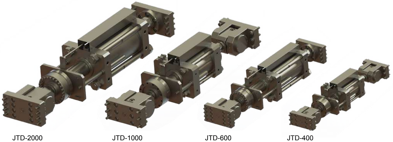
Static Actuators
